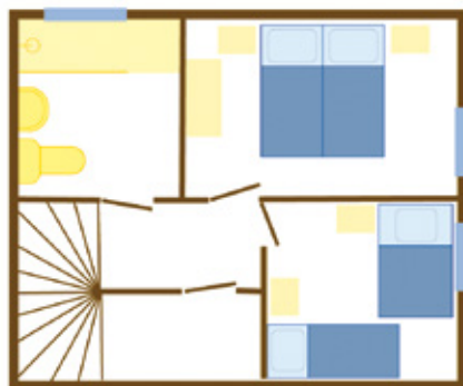
Plattegrond bovenverdieping
